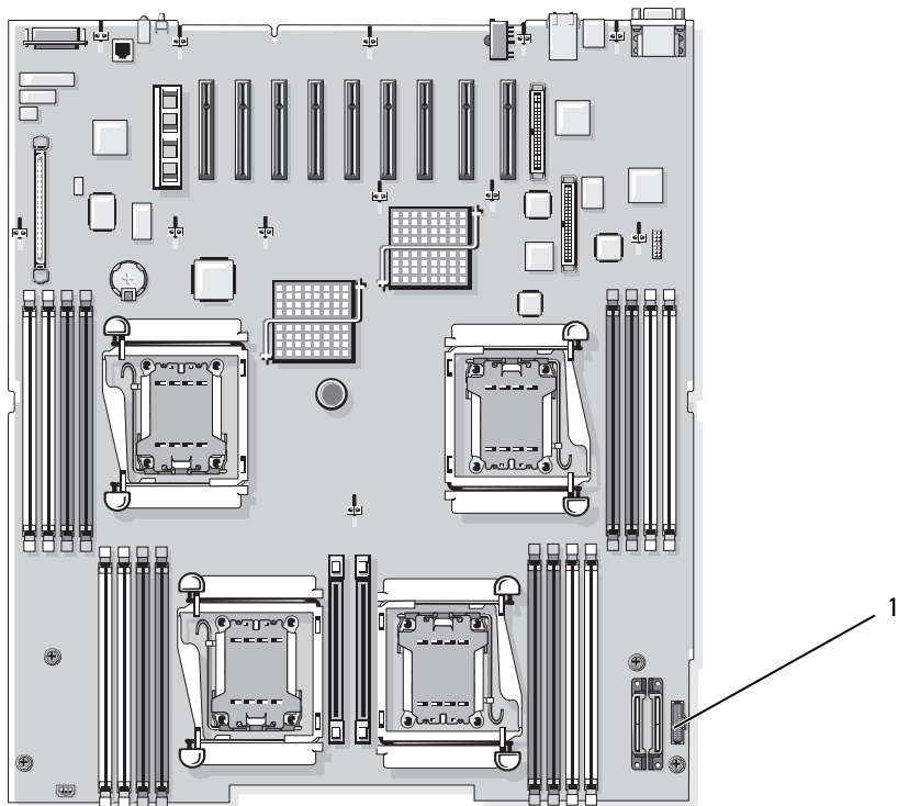
Figura 1. Conector del cable de control de la distribución de alimentación en la placa base
